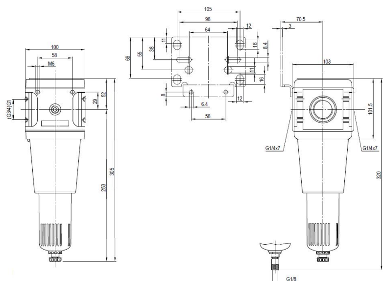
automatisk aftapningsventil
