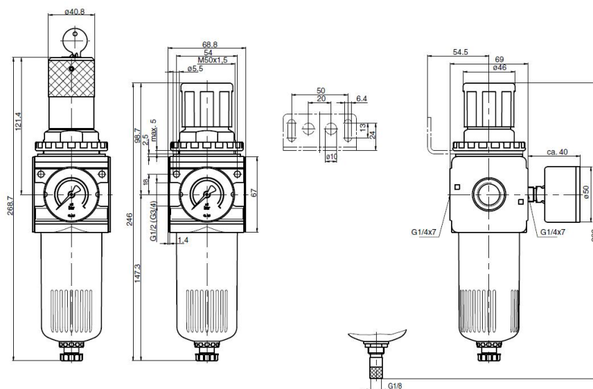
halvautomatiskt avtappningsventil
