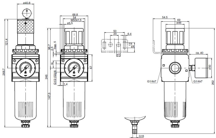
halfautomatische aftapkraan
