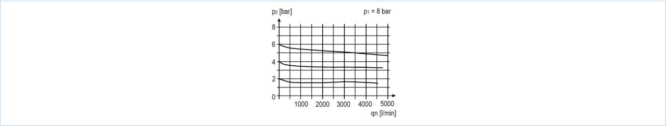
Diagramă de debit pentru domeniul de reglare 0,5...10 bar
