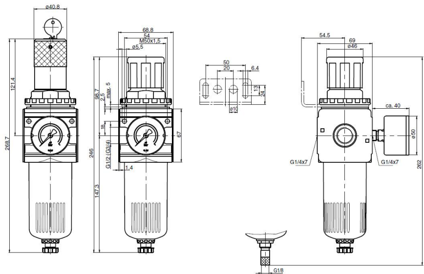
halvautomatisk aftapningsventil
