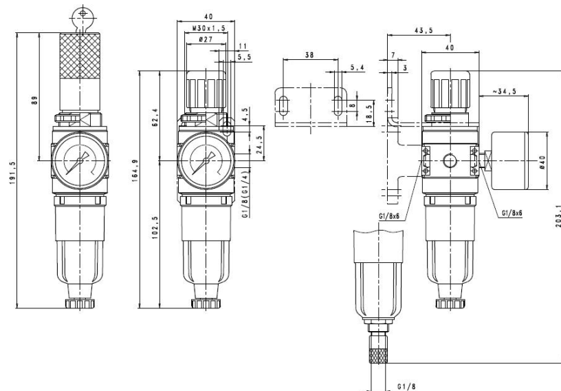
purgeur semi-automatique
