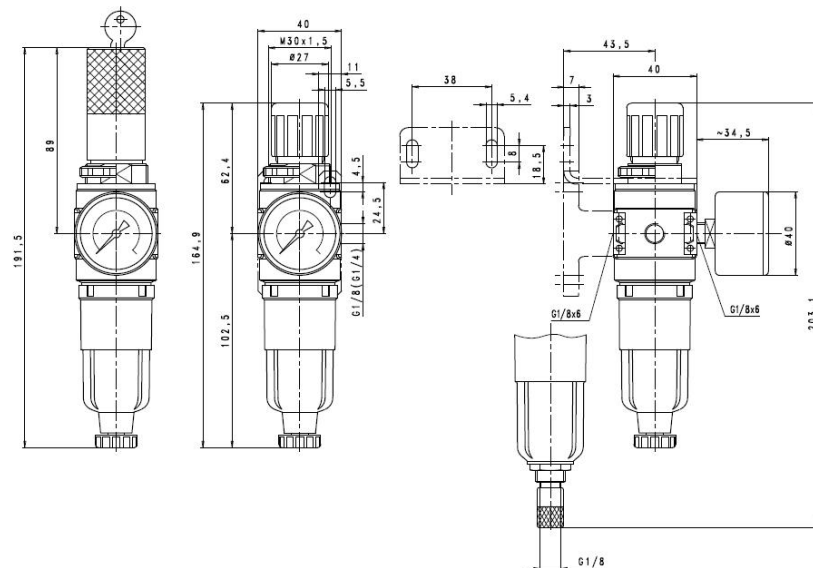
puoliautomaattinen tyhjennysventtiili
