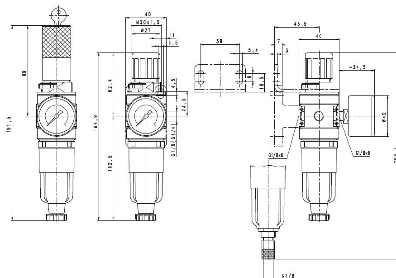
halvautomatisk avtappingsventil
