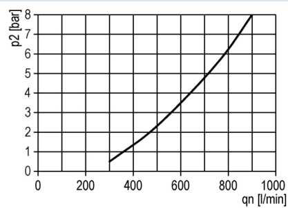
Öljysumuttimen toimintaraja
