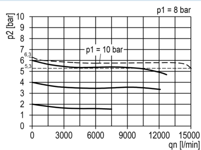
Virtauskaavio
