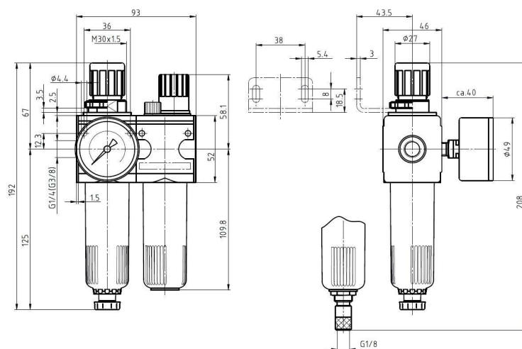
puoliautomaattinen tyhjennysventtiili
