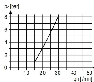
Soglia di intervento dell'oliatore
