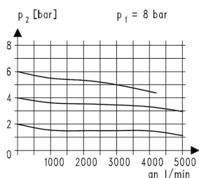
Strömungsdiagramm
