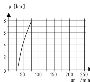
Olieforstøverens aktiveringsgrænse
