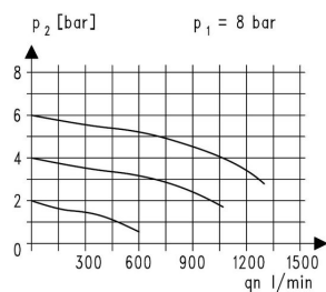
Strömungsdiagramm
