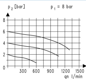
Virtauskaavio
