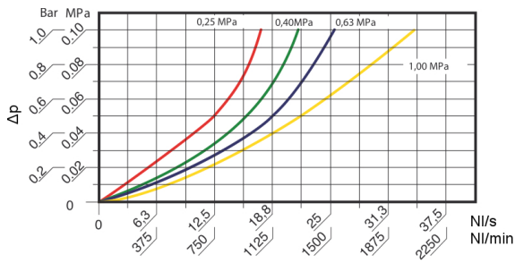
Dijagram prikazuje različite ulazne tlakove do pada tlaka maks. 1bar
