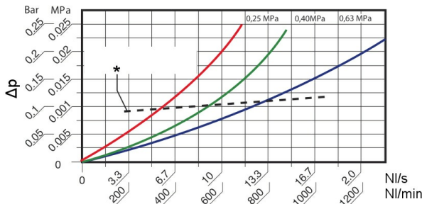
*Rekommenderat maximalt flöde Diagrammet visar olika ingångstryck
