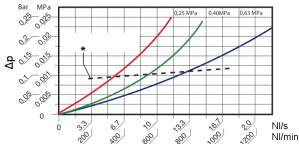
*Aanbevolen maximale doorstroming Het diagram toont verschillende inlaatdrukken
