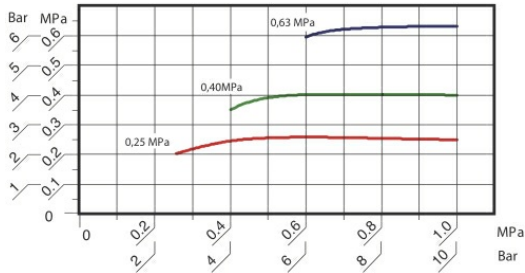
Protok konstantan = 750l/min horizontalna os: Ulazni tlak vertikalna osovina: Izlazni tlak
