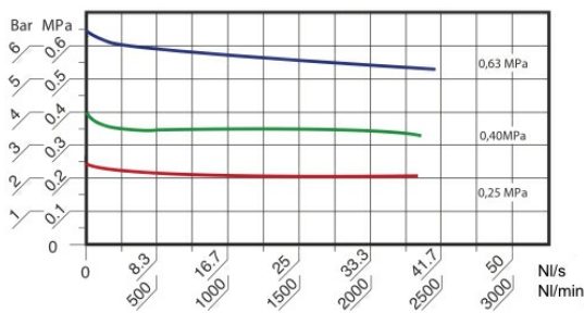
Pression d'entrée = 10bar, Débit en conditions normales
