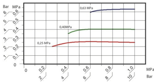
Débit constant = 750l/min axe horizontal: Pression d'entrée axe verticale: Pression de sortie
