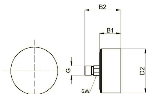
Ø 63 mm
