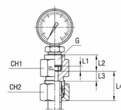
med B3-skæring
