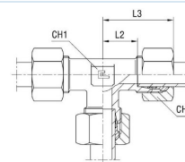
med B3-skæring
