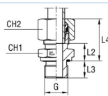
με δακτύλιο κοπής B4-Schneidring
