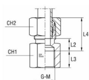
med B3-skjæring
