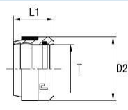
B4-rezalni obroč
