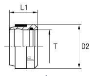
B4-leikkuurengas
