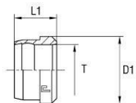
B3-řezný kroužek
