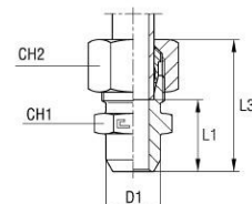
avec bague coupante B3
