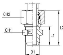
avec bague coupante B4
