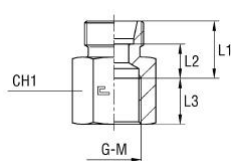
Grundkropp
