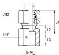
med B4-skärhylsa
