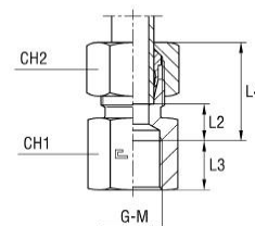
med B3-skjæring
