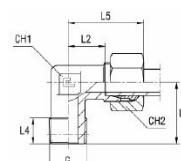
met B3-snijring
