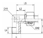
met B3-snijring
