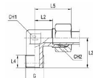
kanssa B3-leikkuurengas
