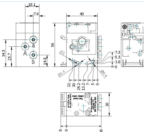
Dimenzijski crtež
