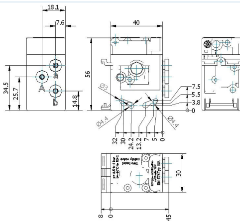
Σχέδιο διαστάσεων
