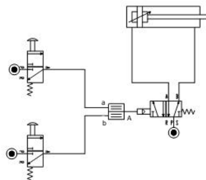
Σχεδιάγραμμα σύνδεσης
