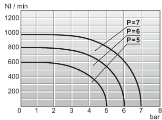
Flödesdiagramm 1/8"
