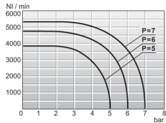
Flödesdiagramm 1/2"
