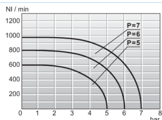
Diagramme de débit 1/8"
