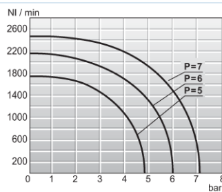
Virtauskaavio 1/4"
