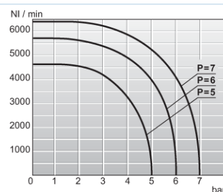
Διάγραμμα ροής 1/2"
