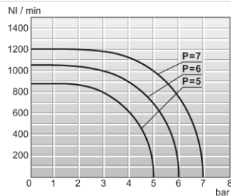
Strømningsdiagramm 1/8"
