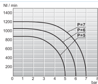
Virtauskaavio 1/8"
