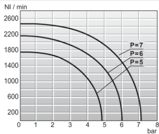
Doorstroombiagramma 1/4"
