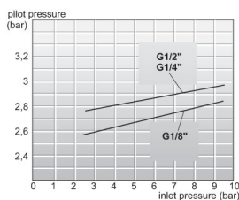
Manövrering pneumatisk/fjäder
