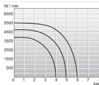
Strømningsdiagramm 1/2"
