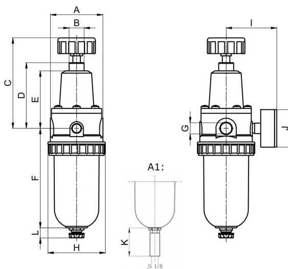
A1: automatikus leeresztőszelep
