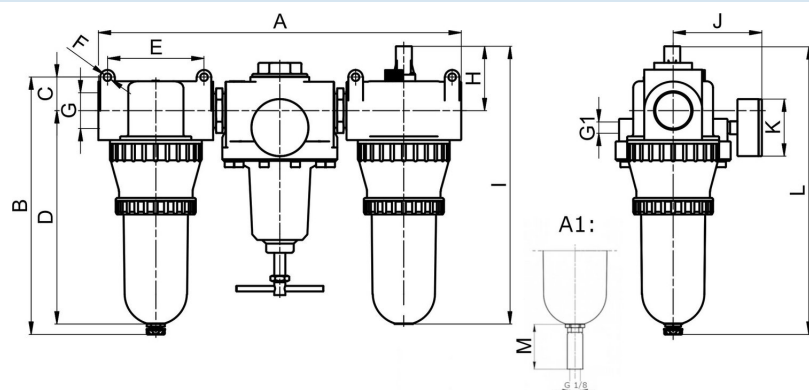
A1: automatski odvodni ventil
