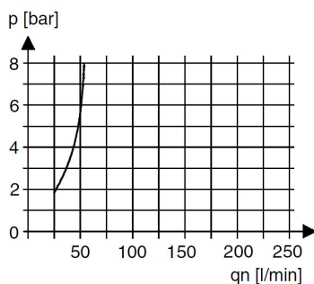
naoljevalnik-meja
