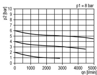
Průtokový diagramm
