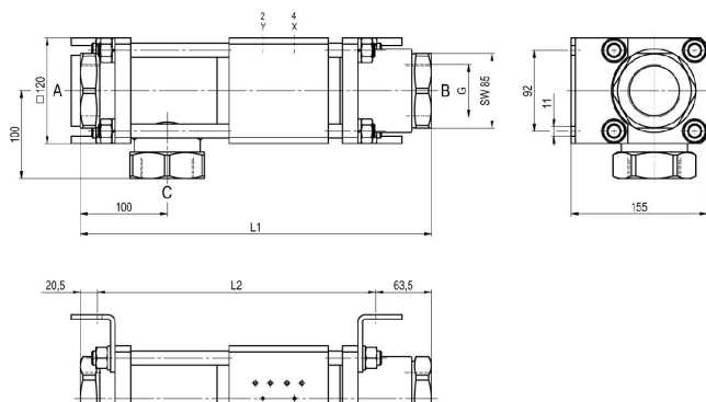
CVTE3-40 Funktion NC
