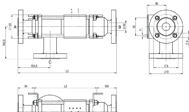
CVFE3-40 Funktion NO
