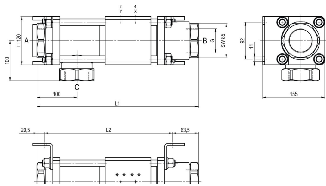
CVTE3-40 Function NC
